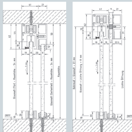
Sturz-/Zwischen-Wand-Montage mit festem Seitenteil (zu 340221)
