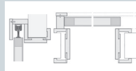
Skizze Variante A: Schiebetürzarge auf Wand
