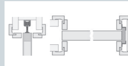
Skizze Variante B: Schiebetürzarge in Wand
